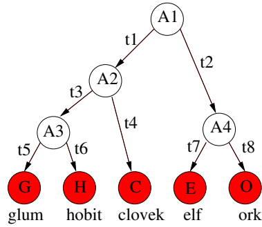
Obr. 3.10: Fylogenetický strom s dĺžkami hrán t_1, \dots, t_8 , s ancestrálnymi bázami A_1, \dots, A_4 a bázami v listoch G, H, C, E, O (ide o označenie neznámých, nie konkrétne hodnoty báz).
