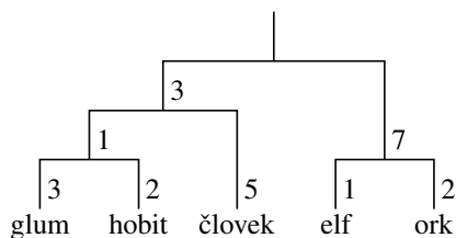
Obr. 3.6: Príklad stromu s dĺžkami hrán a aditívnej tabuľky, ktorá tomuto stromu zodpovedá. Napríklad vzdialenosť hobita a človeka je 8, čo je súčet vzdialenosti 2 medzi hobitom a predkom hobita a gluma, vzdialenosti 1 medzi týmto predkom a predkom hobita, gluma a človeka a vzdialenosti 5 medzi týmto predkom a človekom. Ak máme tabuľku vpravo na vstupe, metóda spájania susedov zrekonštruuje strom naľavo, až na to, že nebude vedieť určiť polohu koreňa.
