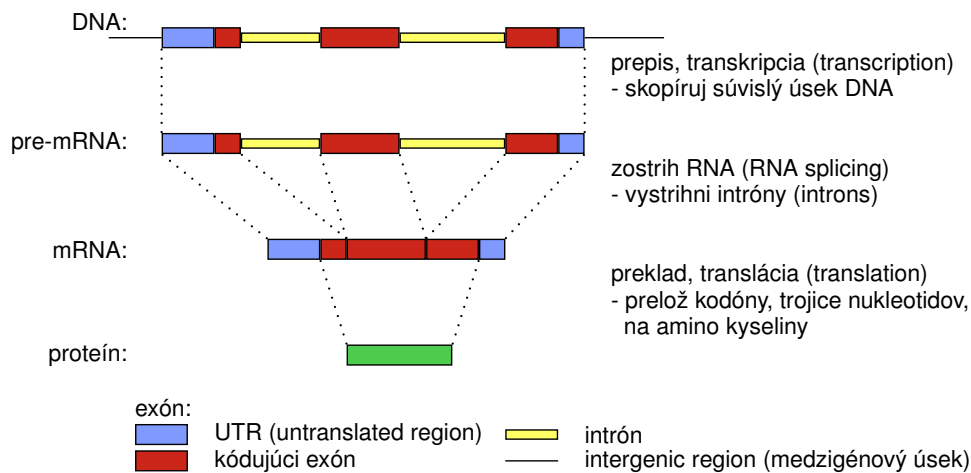
Obr. 4.1: Proces expície génu začína transkripciou z DNA do RNA, z RNA sú vystrihnuté intróny a potom je prekladaná do proteínu.
